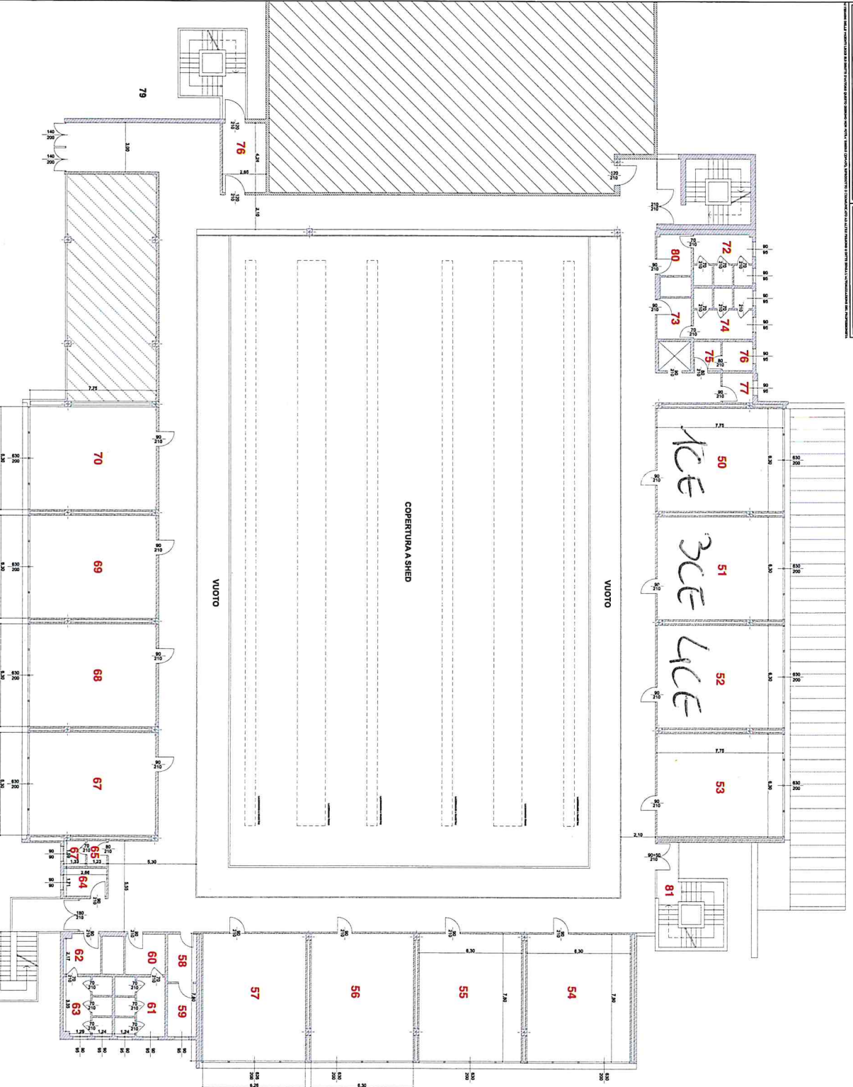
PIANTA PIANO PRIMO - CORPO SCUOLA
